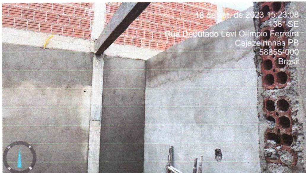
Figura 8 - Execução de chapisco e reboco com fixação de eletrodutos de 25mm.
