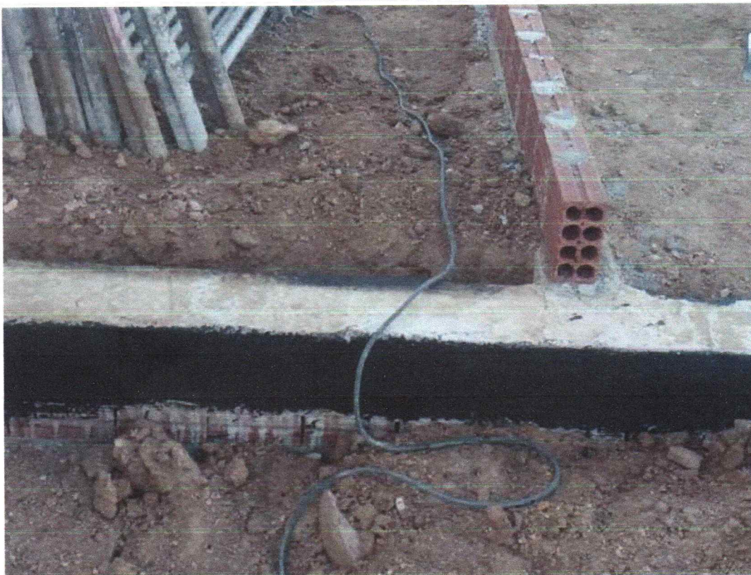
Figura 3 - Impermeabilização de vigas baldrames.
