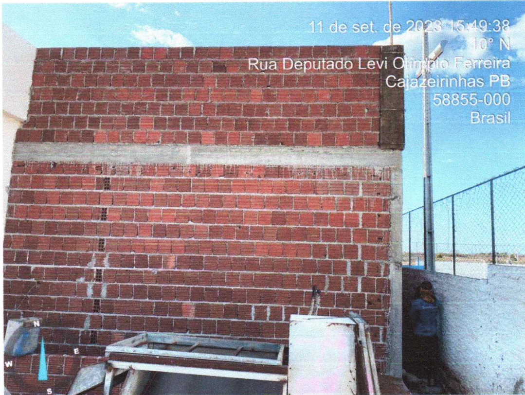
Figura 7 - Execução de alvenaria de vedação e vigas concretadas.
