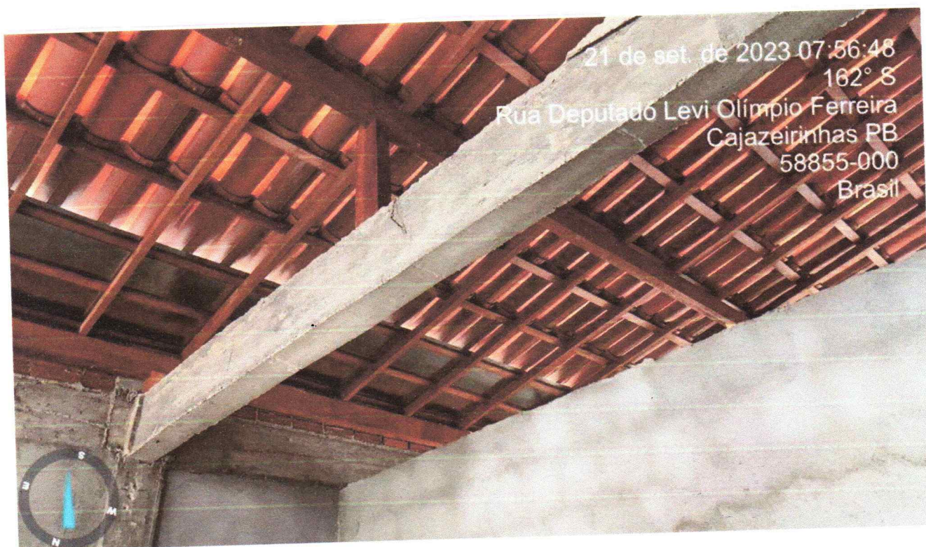
Figura 10 - Execução de coberta e calha.
