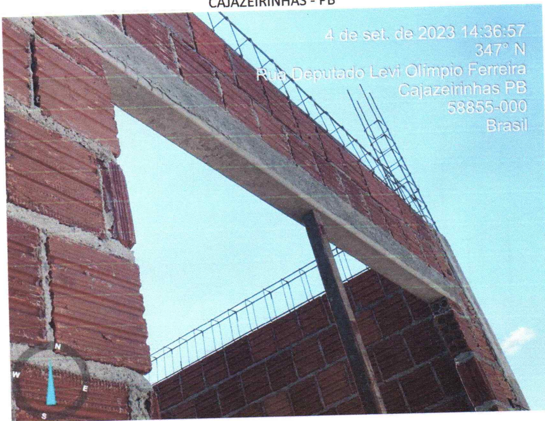
Figura 5 - Execução de vergas e contravergas.
