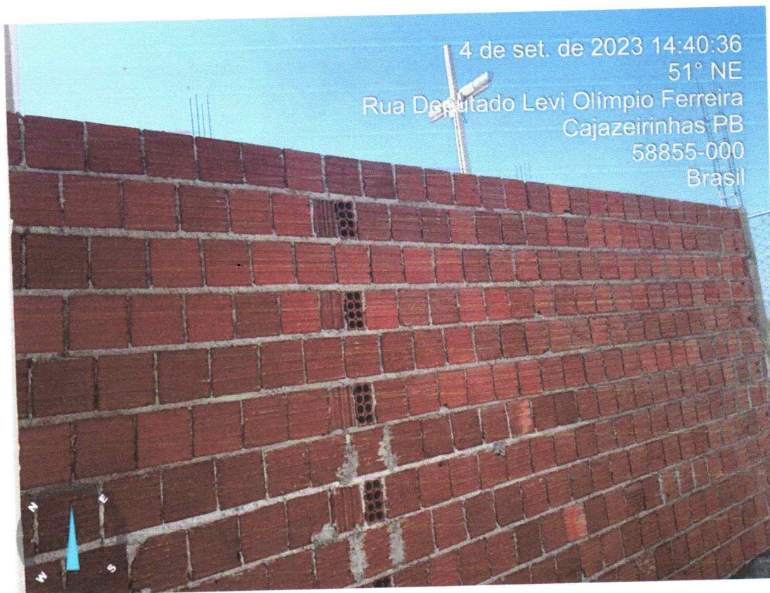
Figura 6 - Execução de alvenaria de vedação.
